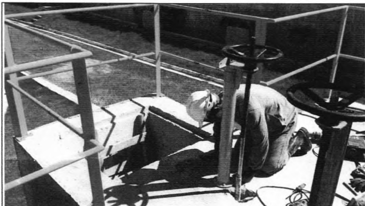
Descrição: Instalação da comporta do extravasor da Caixa de Fluxo 2.
