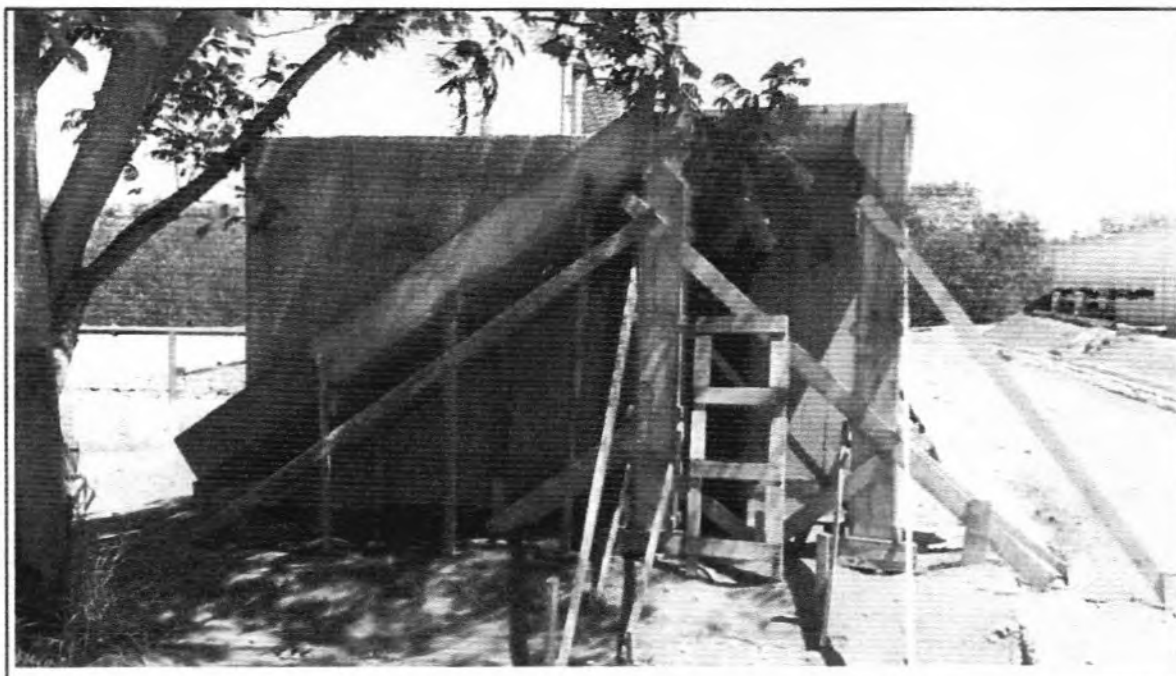
Descrição: Montagem de armadura e forma da escada da Caixa de Fluxo 2.
