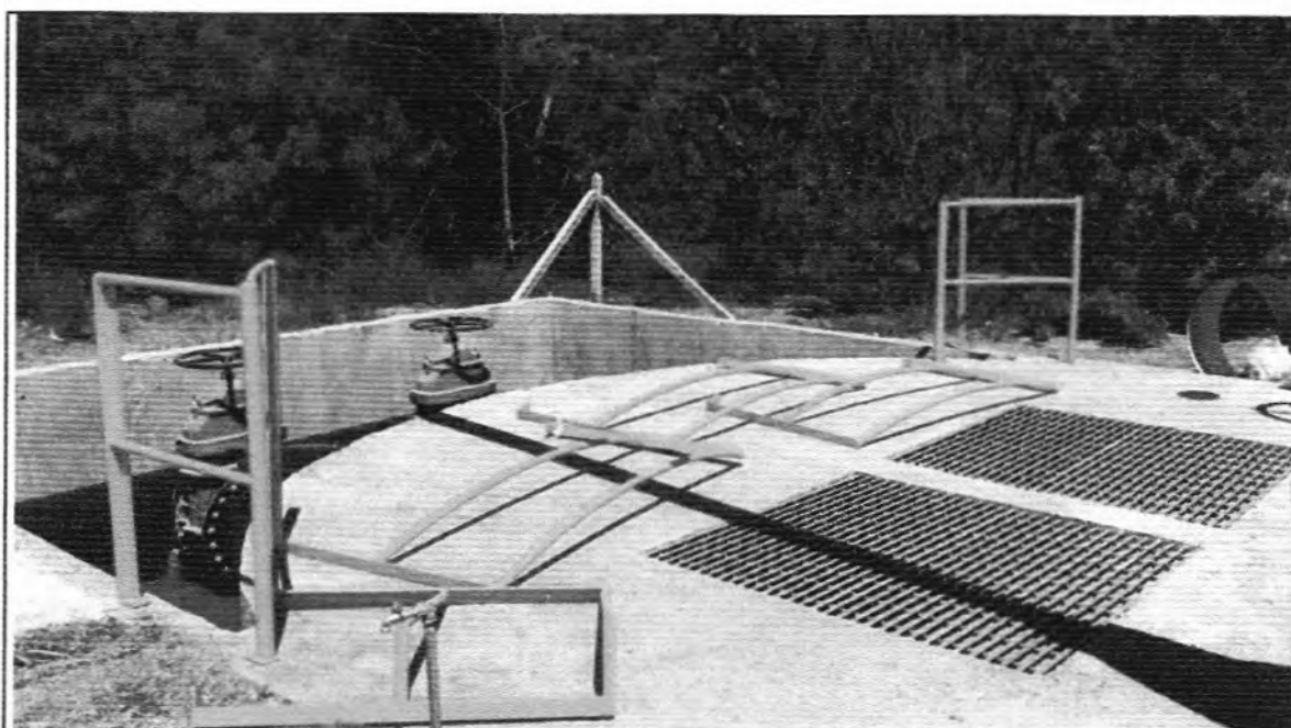
Descrição: Instalação do guarda corpo da EE Final.
